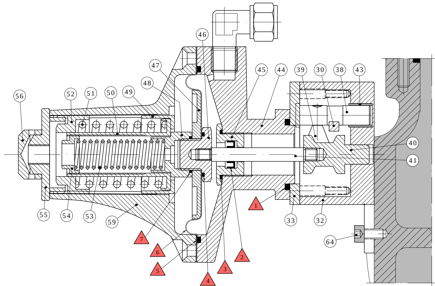
Sezione B-B
