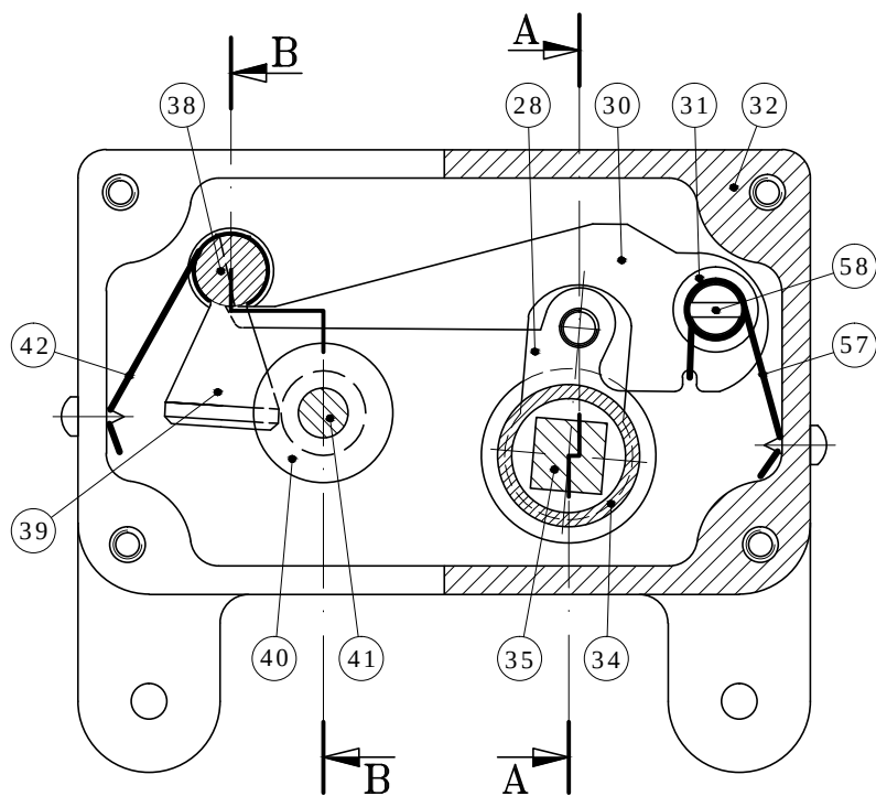
Sezione frontale RELE'
